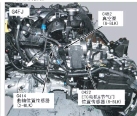
147. 发动机前部
