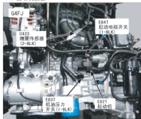
148. 发动机前部
