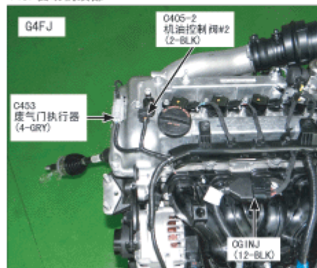
145. 发动机顶部
