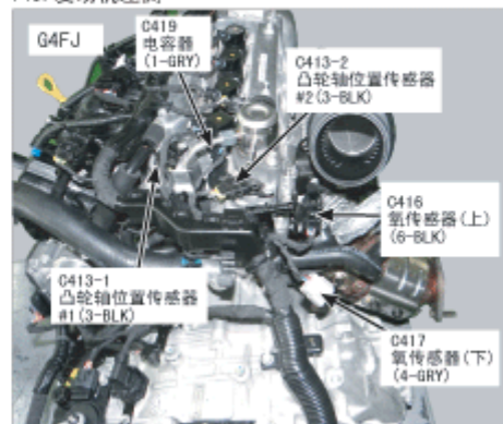
149. 发动机左侧
