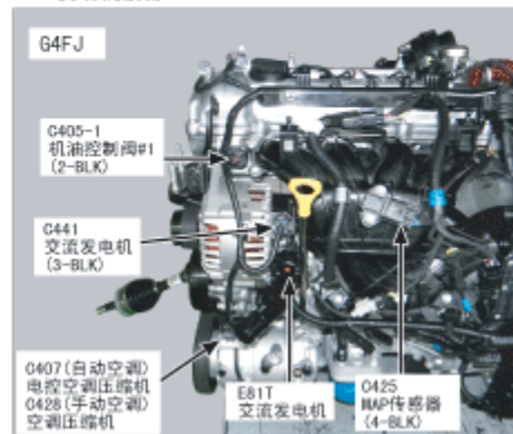
146. 发动机前部
